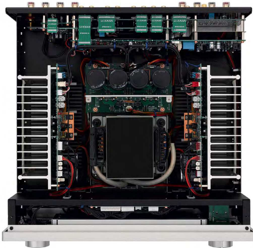
Über dem Trafo sitzen die vier Netzteil-Siebelkos mit jeweils 10.000 µF Kapazität. Vorne rechts, unscheinbar, aber aufwendig: der prozessorgesteuerte Pegelregler mit Spannungsteilern aus Festwiderständen.
